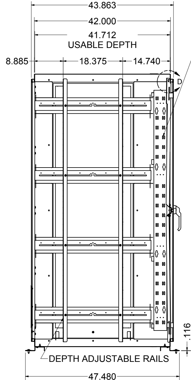
SECTION A-A
